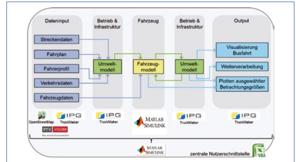
Abbildung 36: Struktur des Simulationsmodells zur Abbildung des Gesamtsystems
