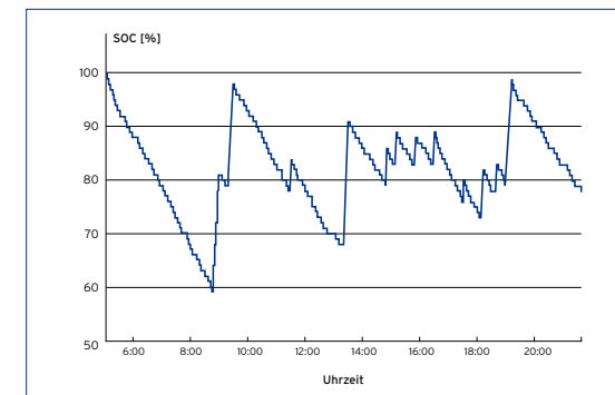
Abbildung 41: SOC-Verlauf Traktionsbatterie über einen Tag
