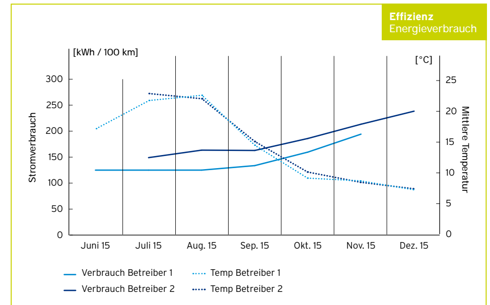
Abbildung 18: Batteriebus mit elektrischer Heizung - Betrachtung Energieverbrauch
