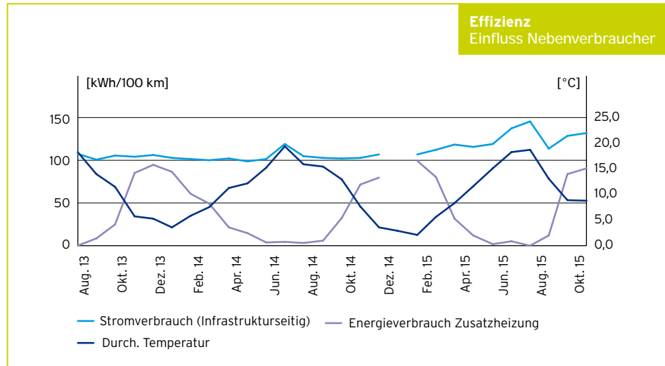
Abbildung 17: Batteriebus mit Dieselsatzheizung - Betrachtung Energieverbrauch für Fahrtrieb und Heizung Fahrgastraum
